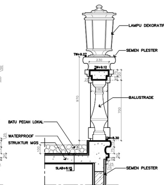
1D POTONGAN 2 SKALA 1 : 15
