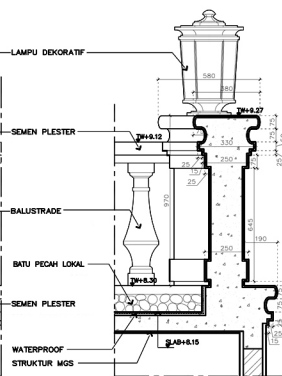
1C POTONGAN 1 SKALA 1 : 15
